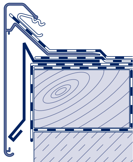
Sanierung auf vorhandener Windfeder
