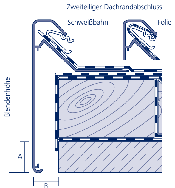
Sanierung auf vorhandener Windfeder
